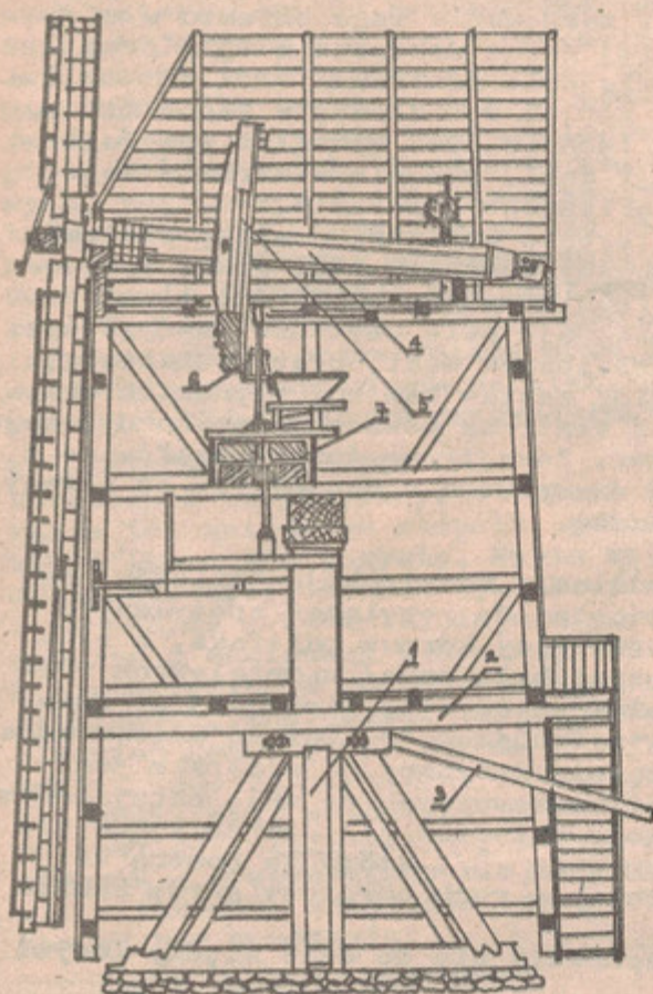
Rys.1. Ogólna konstrukcja koźlaka
