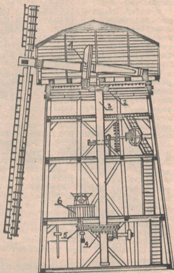
Rys.2 Konstrukcja wiatraka typu paltrak
